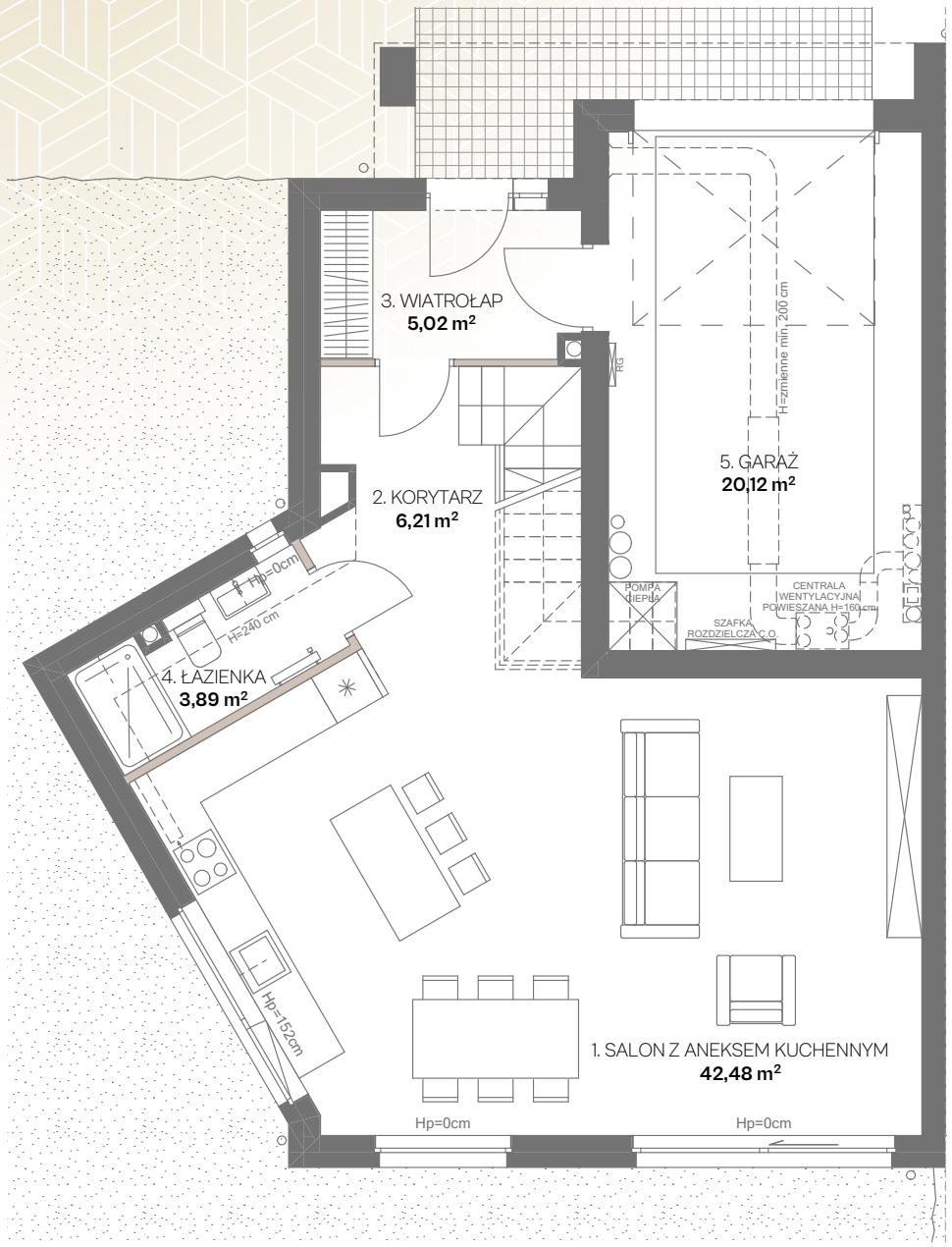
RZUT PARTERU
