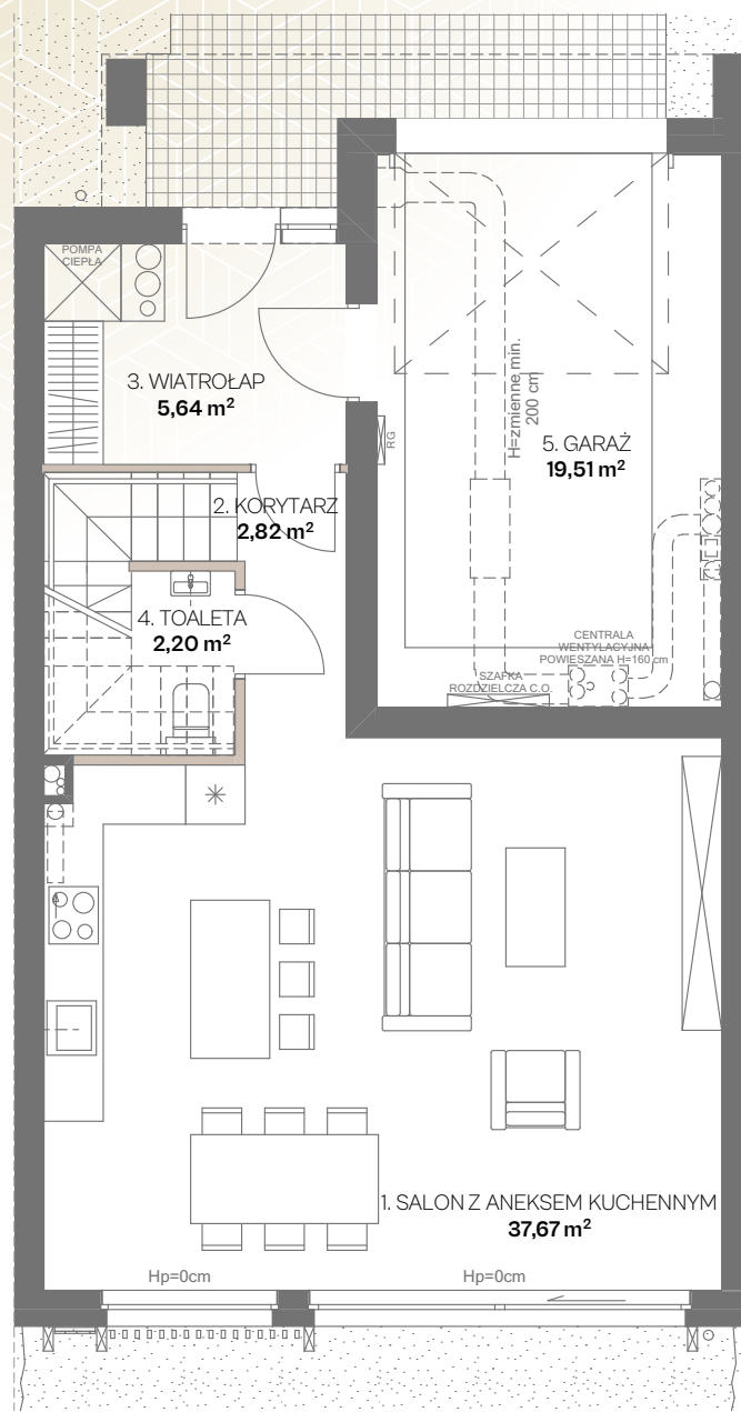
RZUT PARTERU
