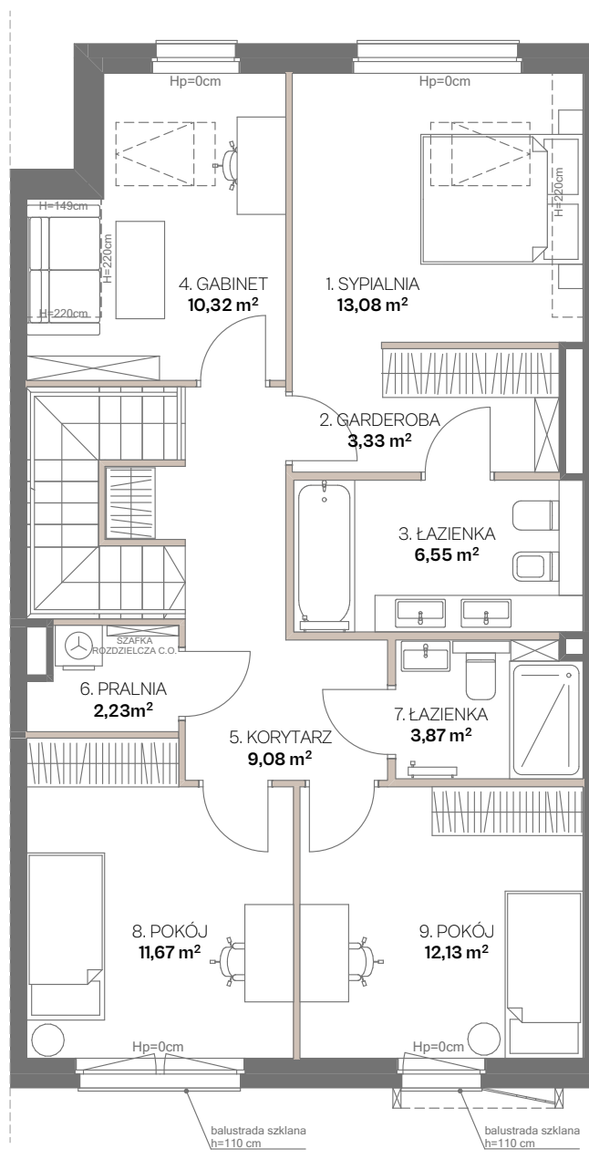
RZUT 1. PIĘTRA
