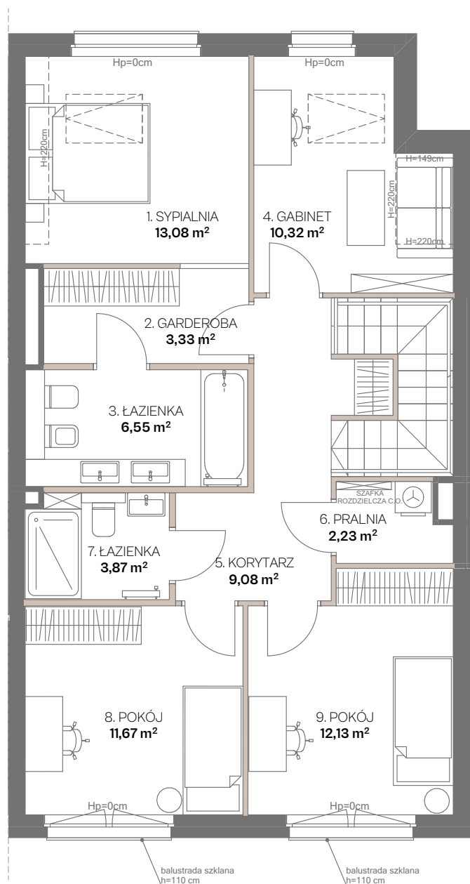
RZUT 1. PIĘTRA
