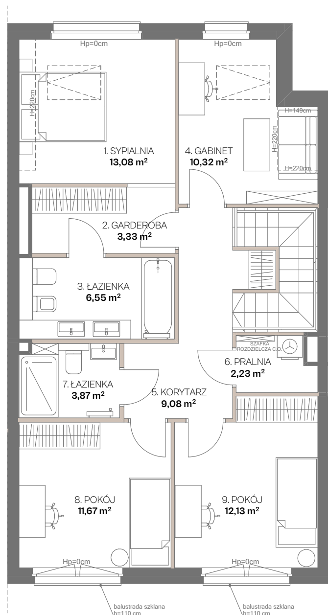
RZUT 1. PIĘTRA
